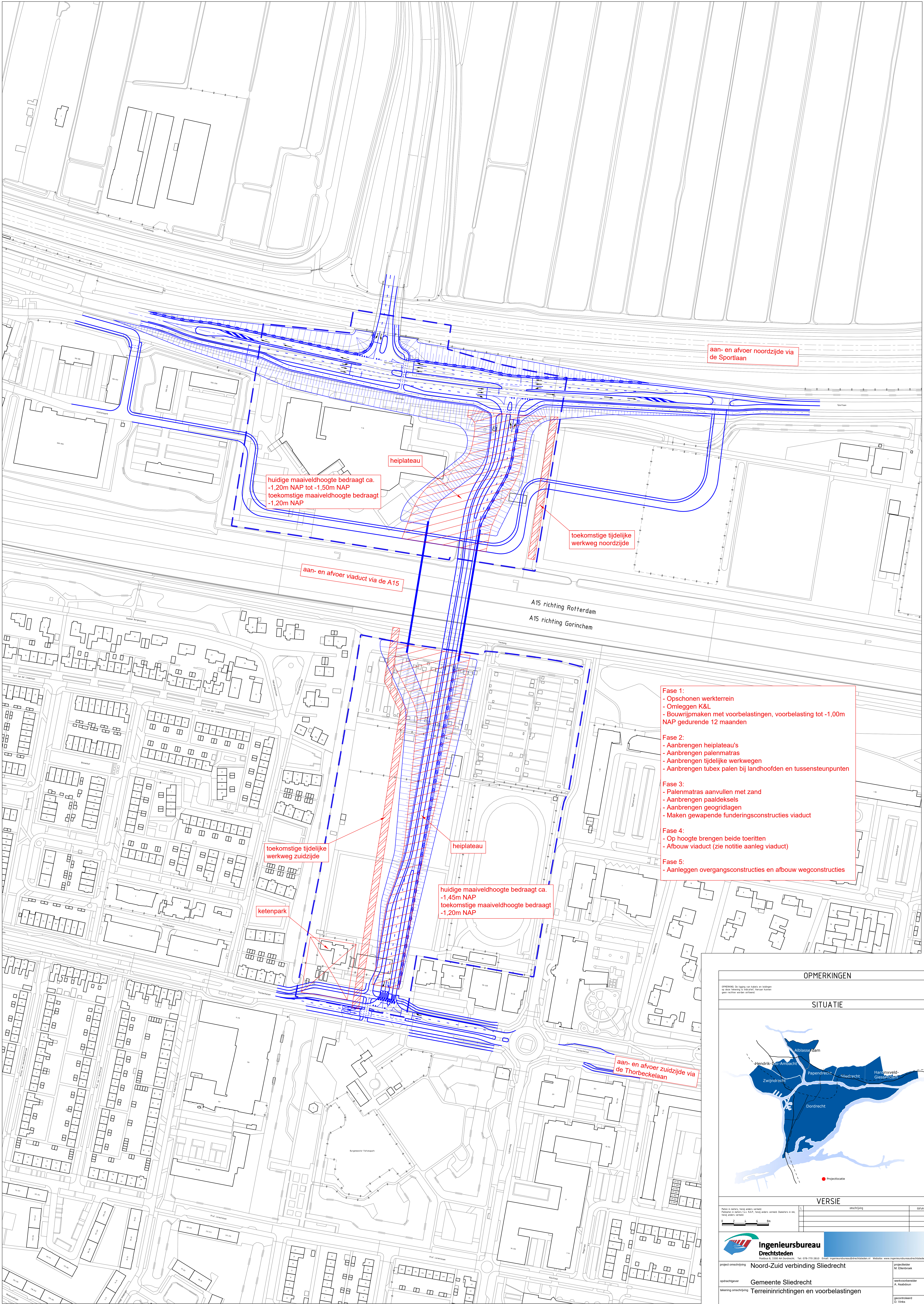
Situatie SCHAAL 1 : 1000
